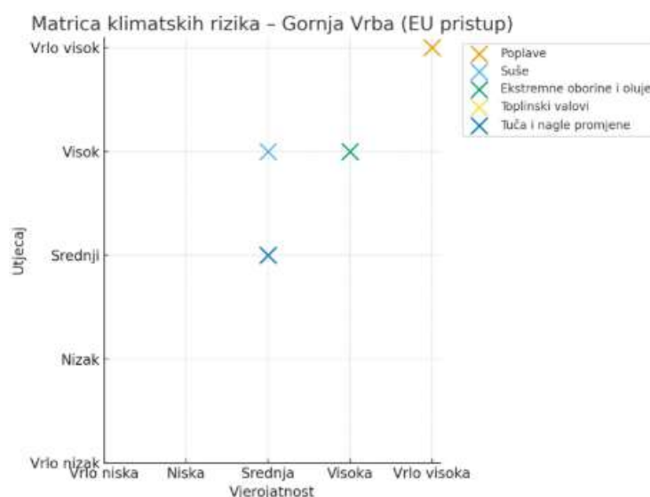
Slika 2: Klimatski rizici na području Općine
